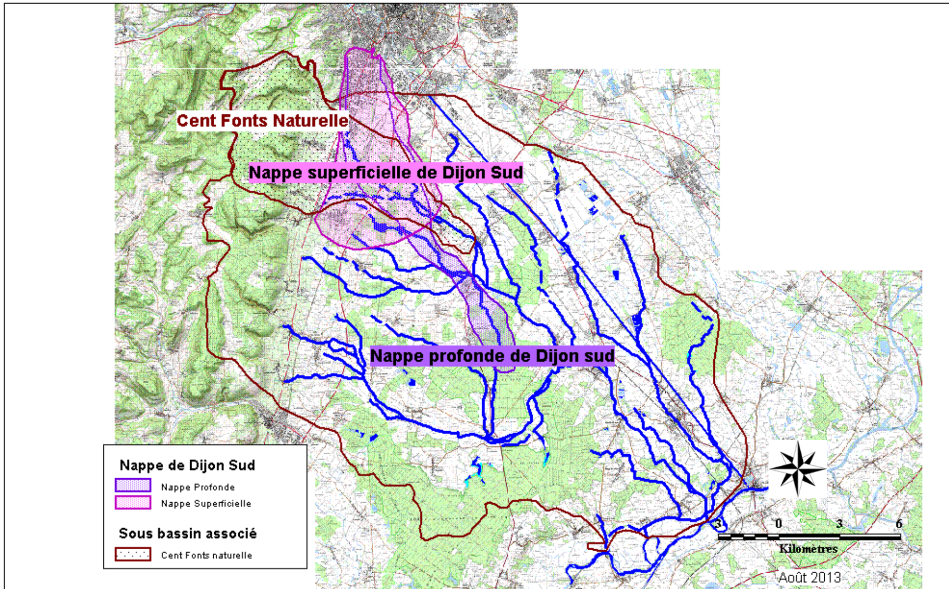
CARTE 6 : MASSE D'EAU NAPPE DE DIJON SUD / CENT FONTS NATURELLE
